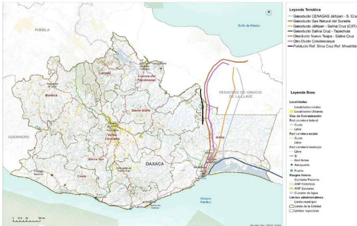
Mapa 86. Ductos en el estado de Oaxaca.
