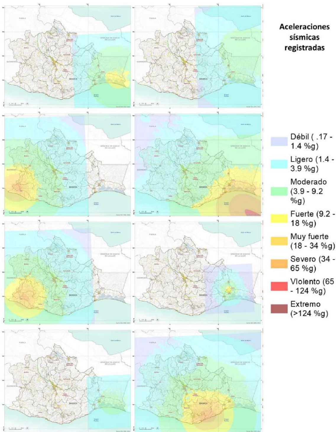
Mapa 28. Aceleraciones sísmicas.
