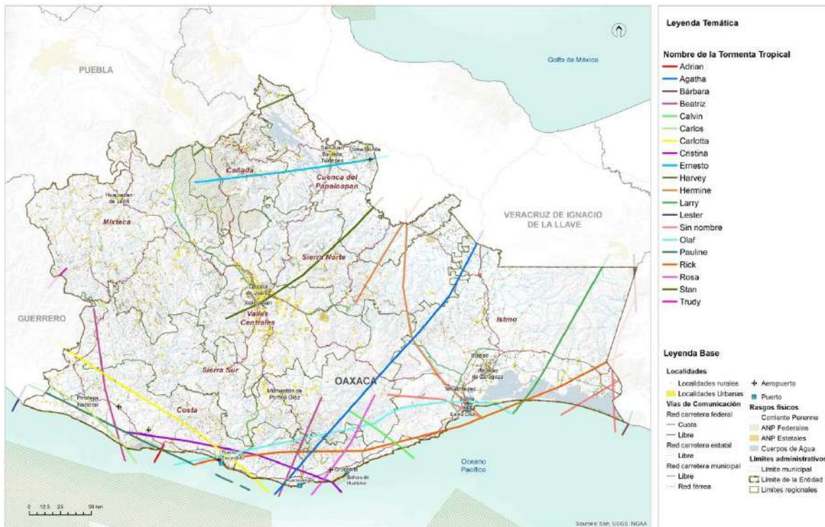
Mapa 34. Trayectoria de tormentas tropicales, 2010-2023.
