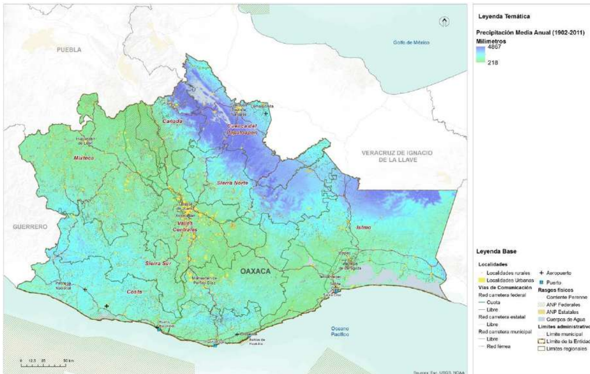
Mapa 10. Precipitación media anual en el estado de Oaxaca (periodo de 1902 a 2011).
