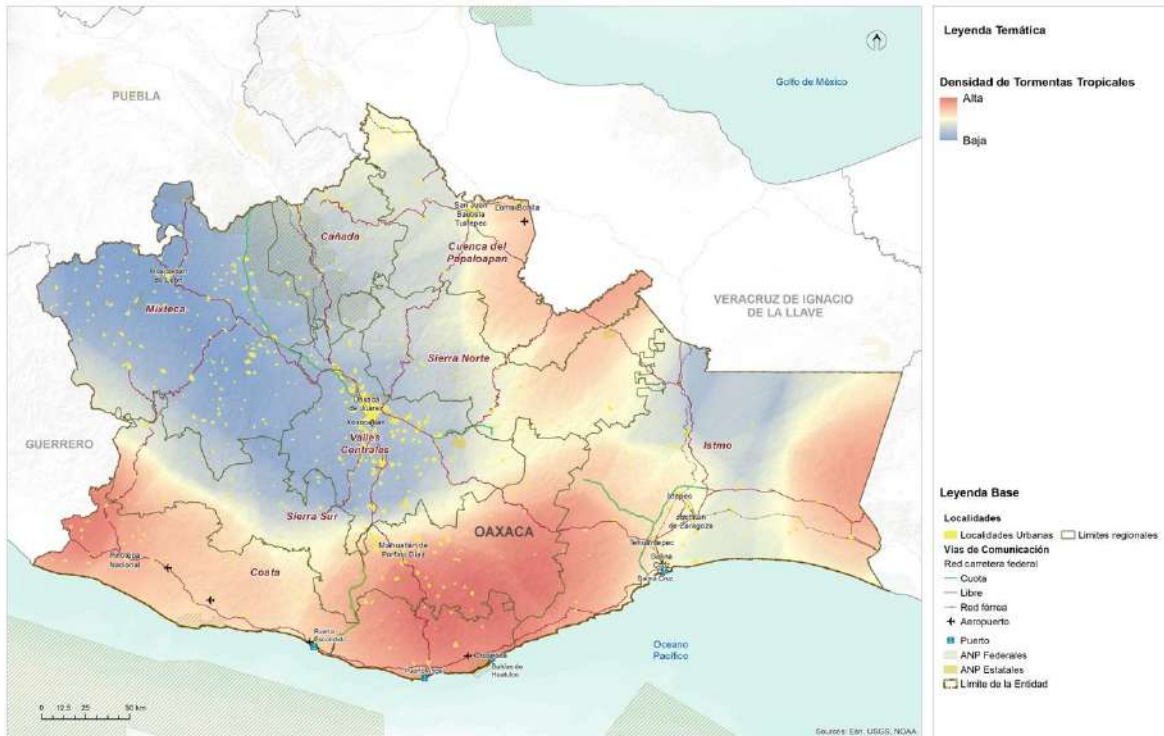
Mapa 37. Densidad de tormentas tropicales, 1980-2023.
