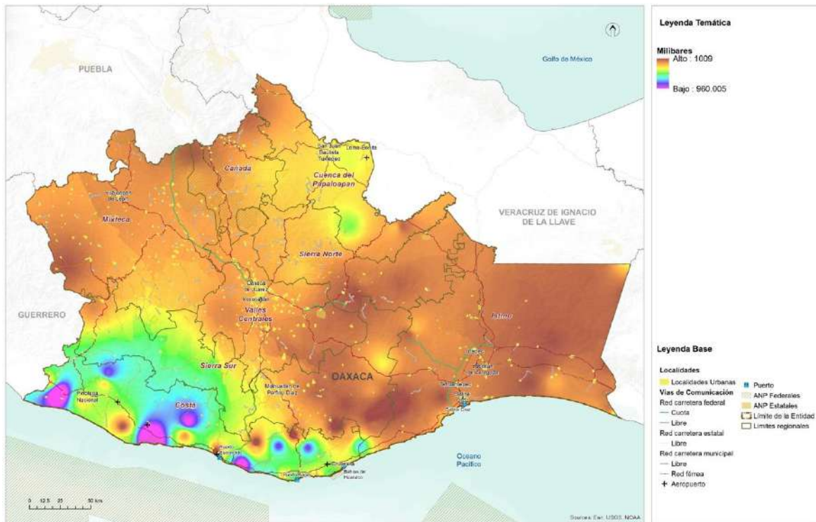
Mapa 35. Presión barométrica.
