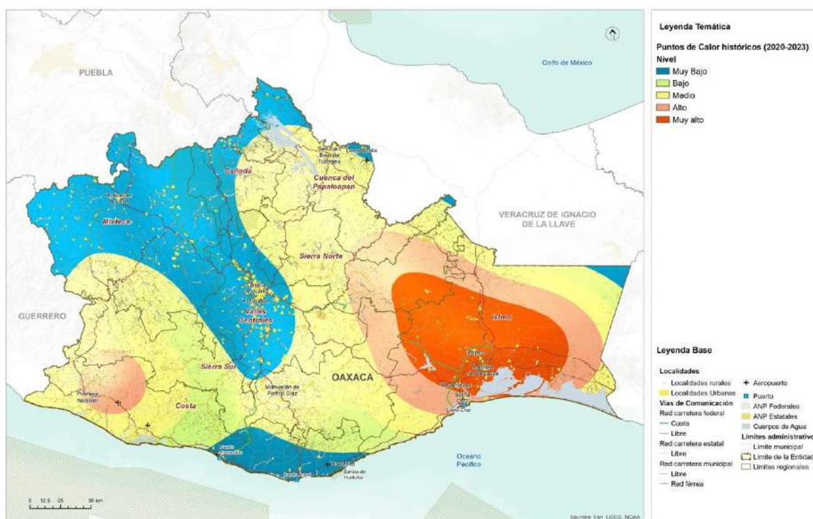
Mapa 26. Puntos de calor históricos en el estado de Oaxaca.
