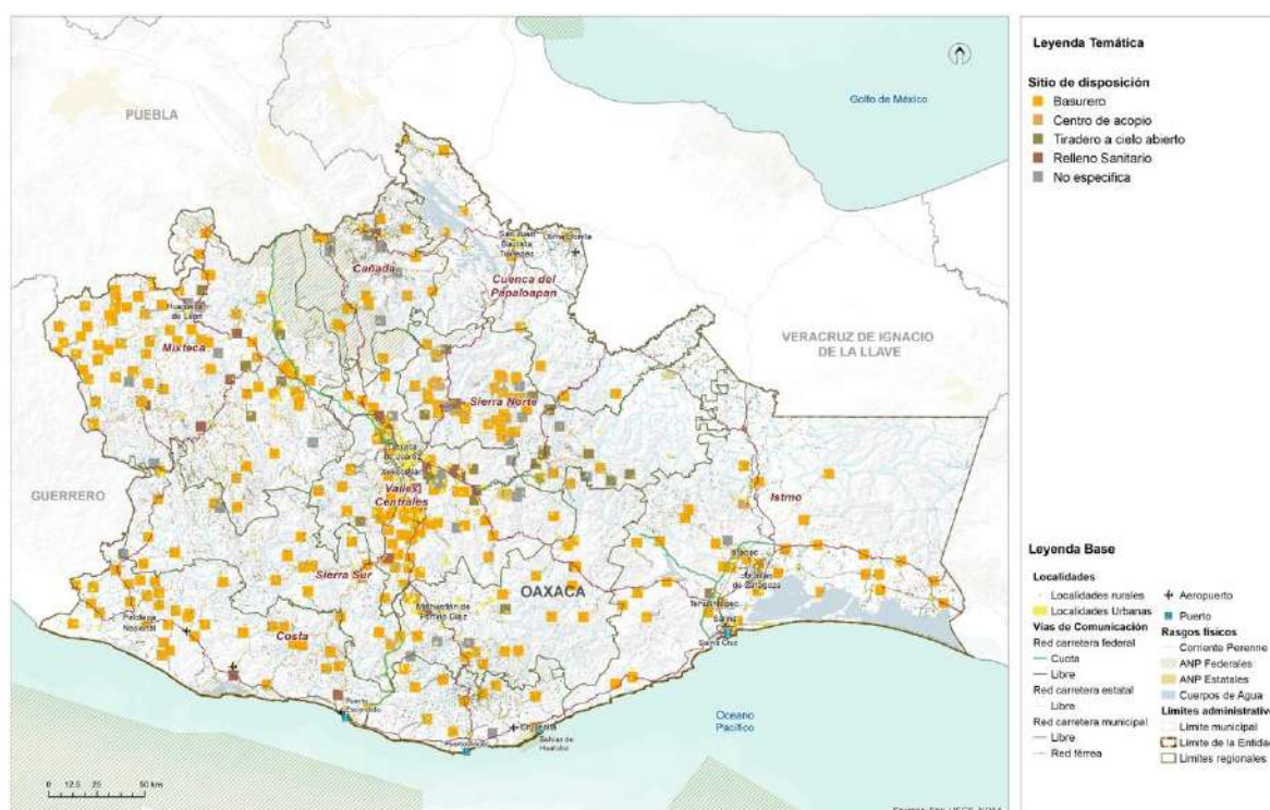
Mapa 24. Ubicación de los sitios en donde se disponen los residuos sólidos.
