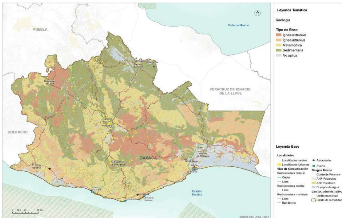
Mapa 2. Tipos de rocas.
