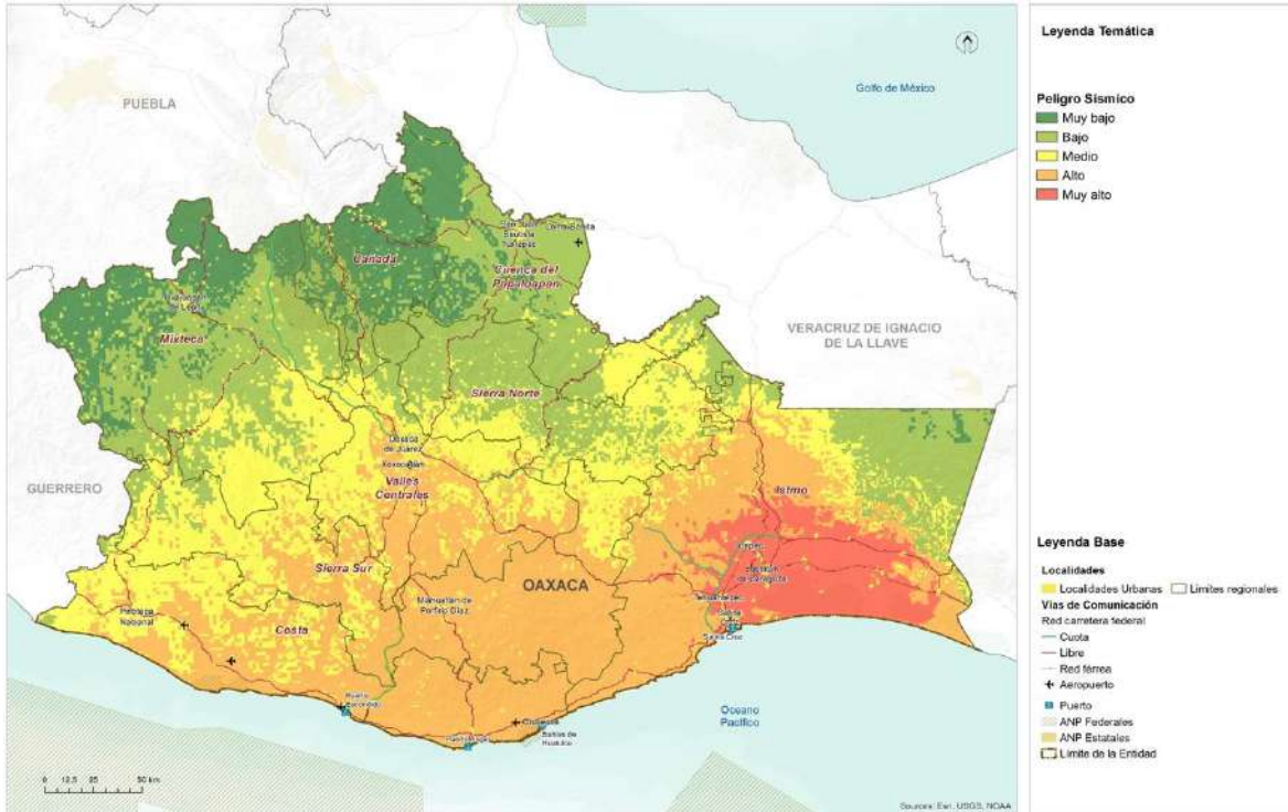
Mapa 29. Peligro sísmico.
