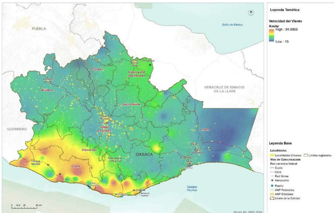
Mapa 36. Velocidad del viento.
