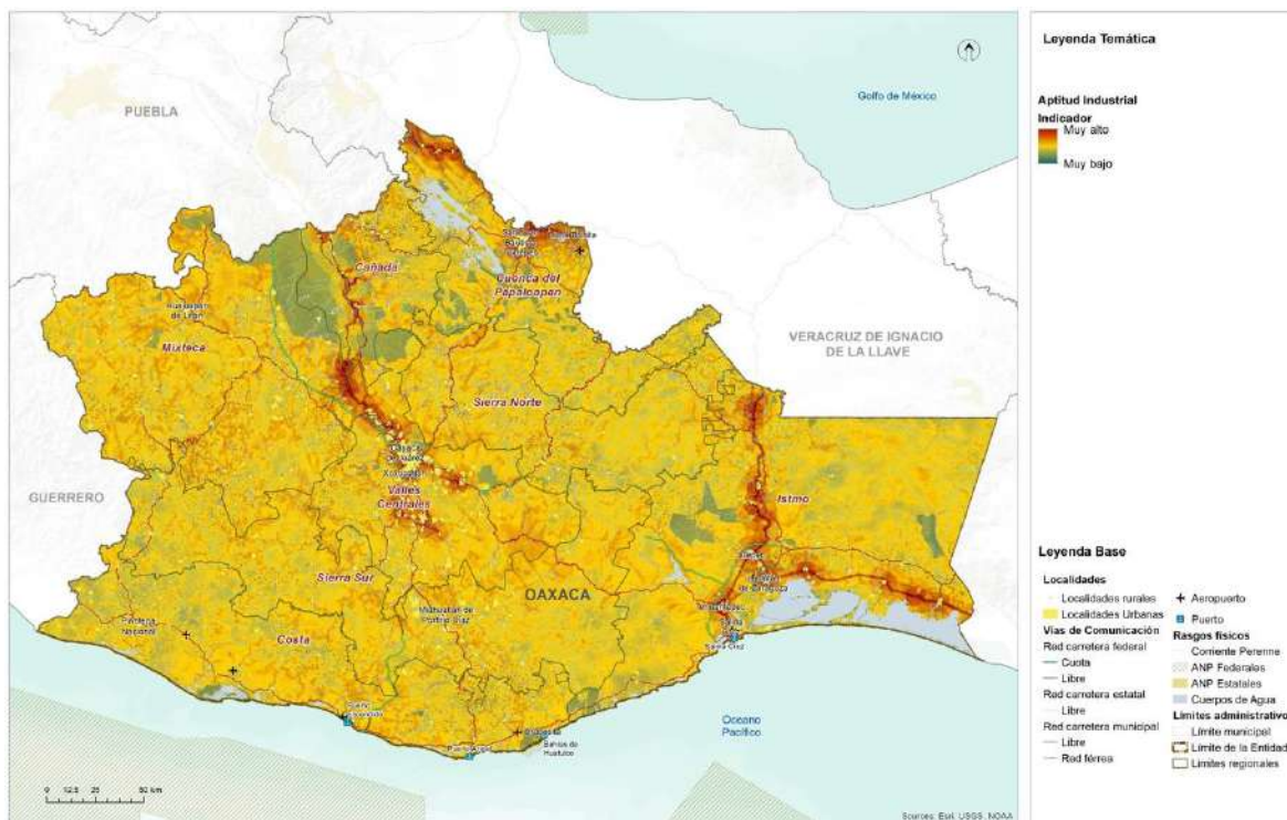
Mapa 117. Aptitud territorial para desarrollo industrial.
