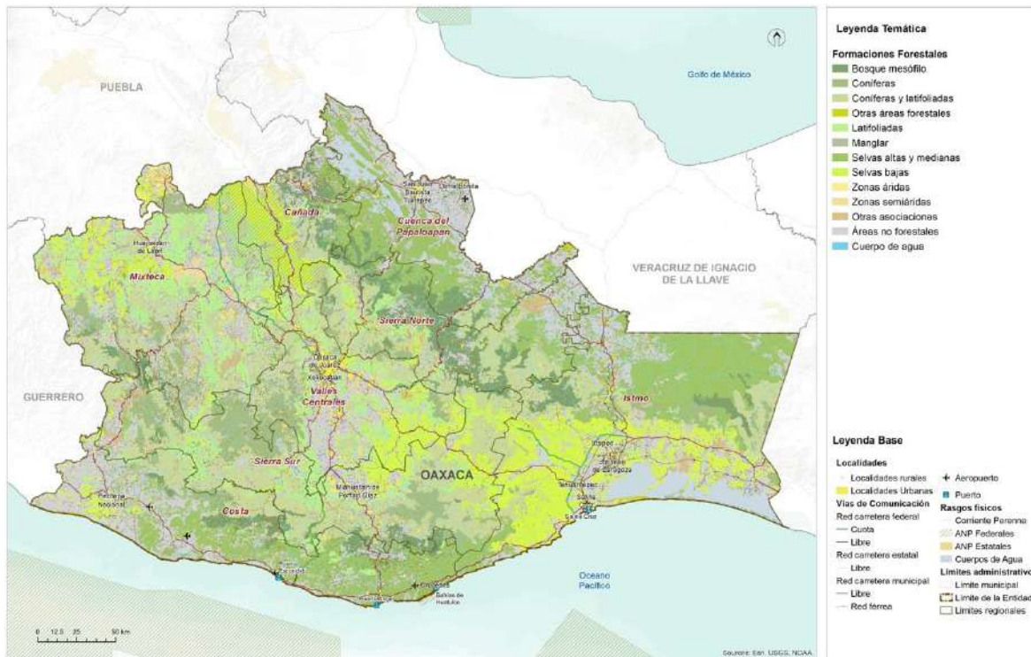
Mapa 19. Formaciones forestales.
