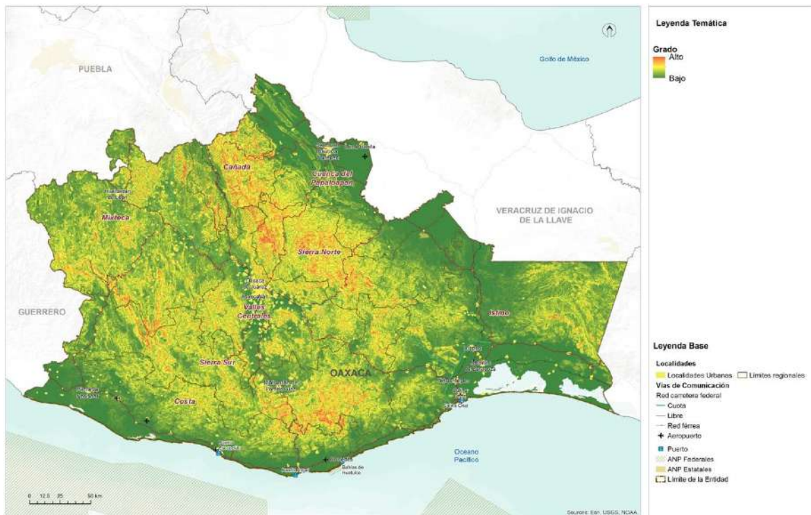
Mapa 30. Susceptibilidad a la inestabilidad de laderas.
