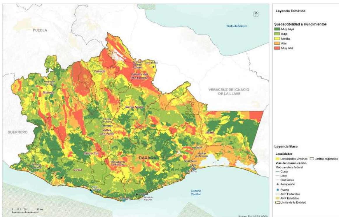
Mapa 33. Susceptibilidad a hundimientos.
